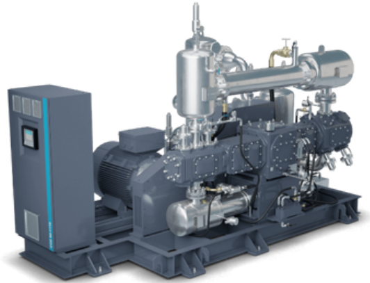
CO2 Centrifugal Compressor
